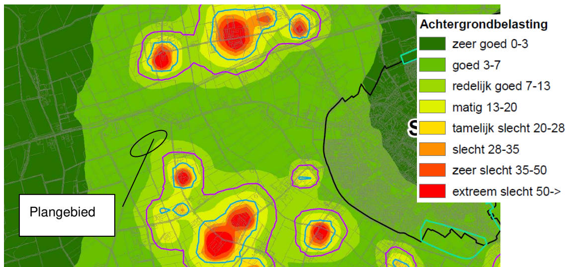
Figuur 33: Achtergrondbelasting ter plaatse van de omgeving van het plangebied
