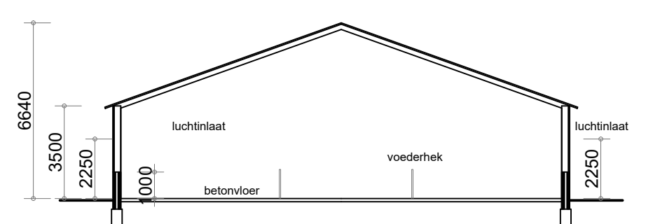
- Doorsnede B - B gebouw 3 -
