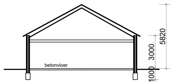
- Doorsnede A - A gebouw 2 -
